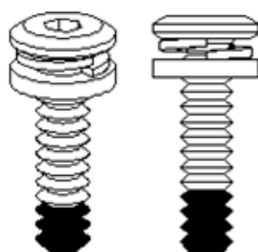
M6x25mm 4x
