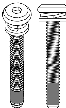
M6x39mm 16x
