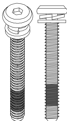
M6x42mm 4x
