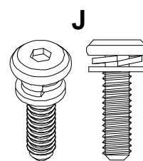
M6x15mm 12x
