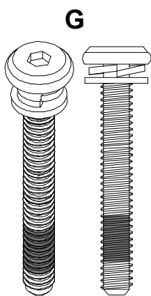
M6x40mm 12x
